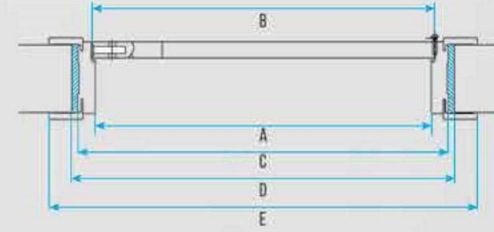
RESİM 1: KAPI GENEL KESİTİ
