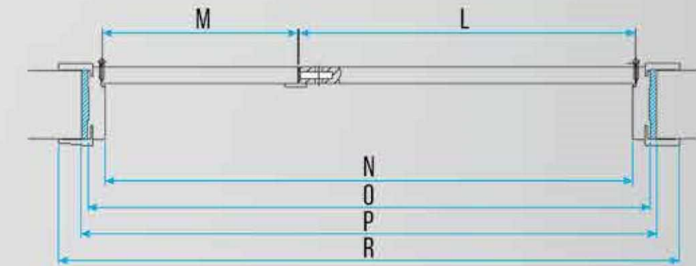
RESİM 3: SALON KAPISI GENEL KESİTİ
