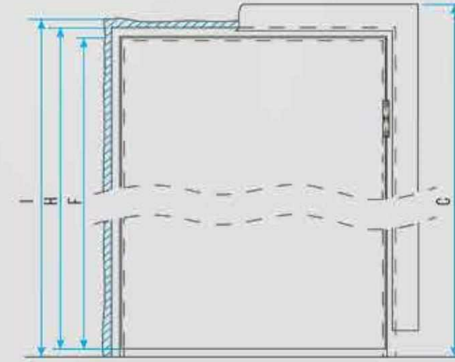
RESİM 2: KAPI YÜKSEKLİKLERİ
